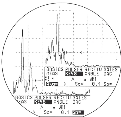
超音波検査 内面割れ調査
